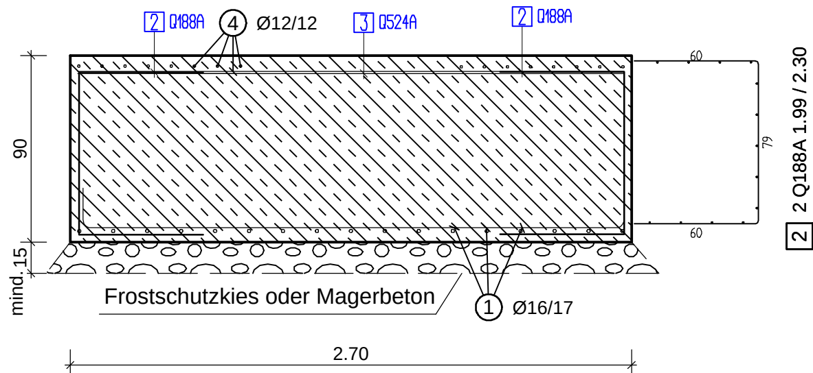
Schnitt 1 - 1 M. 1 : 25
