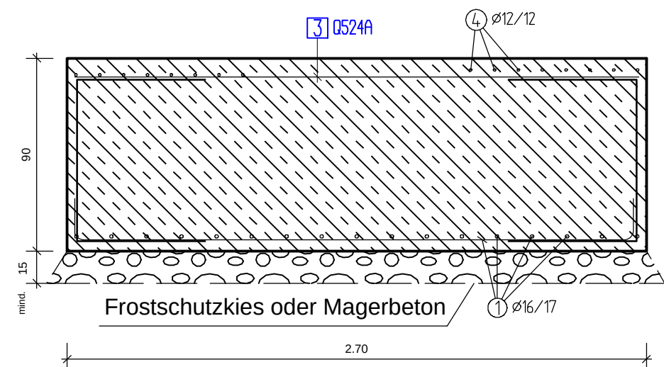
Schnitt 2 - 2 M. 1 : 25
